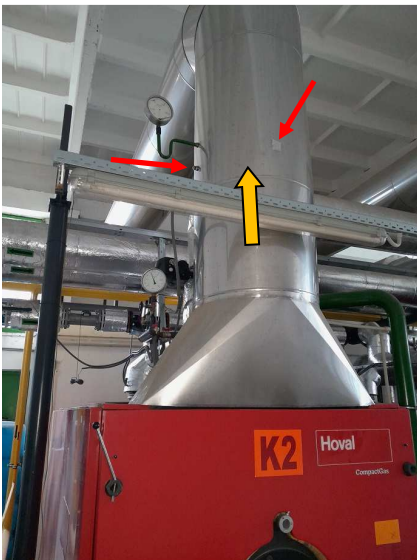
▲ Obrázok č. 3 Miesto merania kotla K2 ← a smer prúdenia spalín ←
